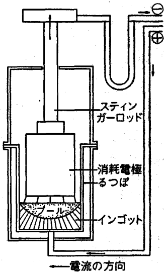
図 2 同軸型 Consel-VAR
