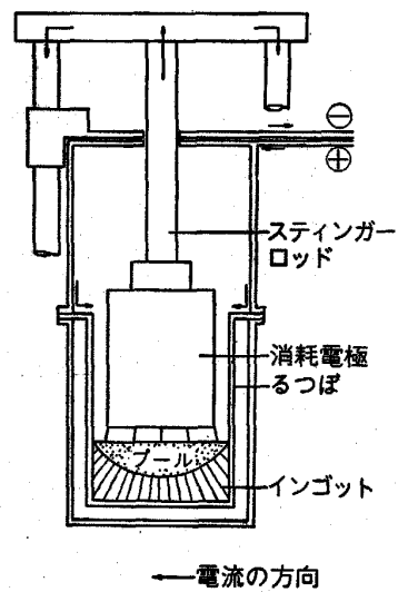
図 2 同軸型 Consel-VAR
