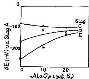
図2. 塩基度に対する Al_2O_3 添加の影響
