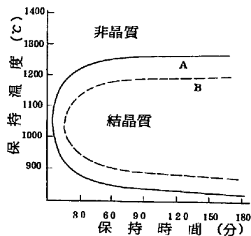
図1 恒温変態曲線
