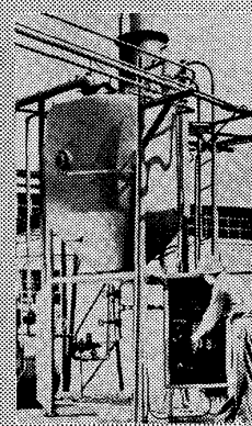
液中燃焼装置
