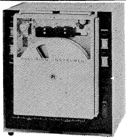
PI-207型 7チャンネル 磁気テープ・レコーダ 超小型 (約40×47×25cm) 軽 量 (約30kg)
