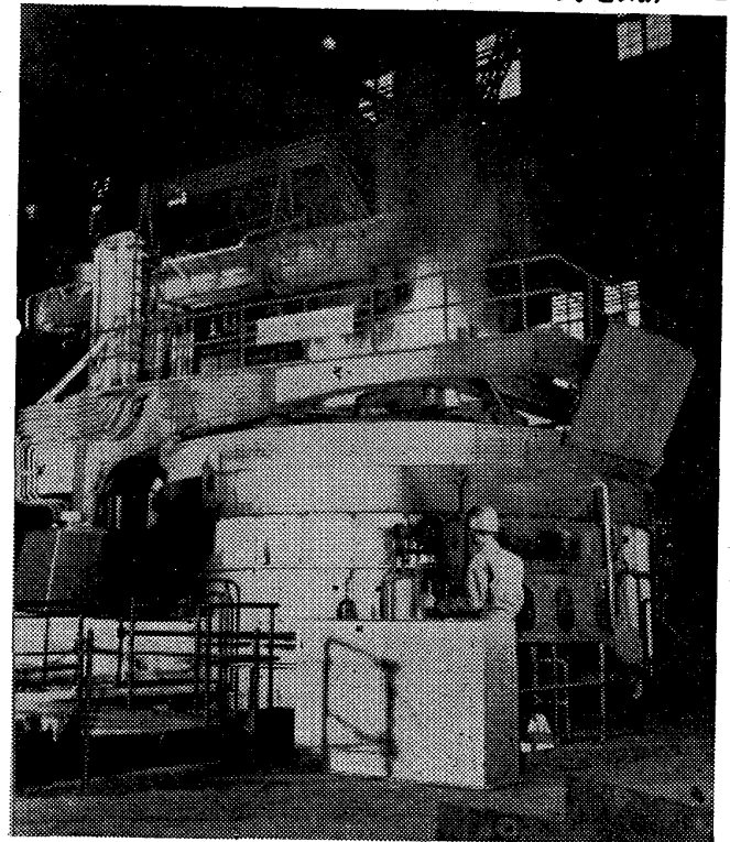
80t B. B. C. - KRUPP 式電気炉
