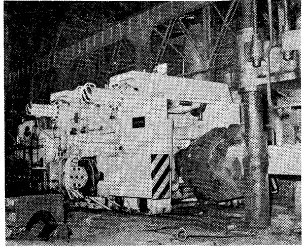
軌道走行式
