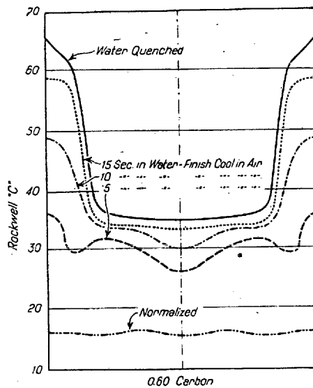
第1圖 C 0.6% 1 回焼入法
