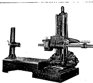
1/4 吋水平シヤ・ボーリングマシン
