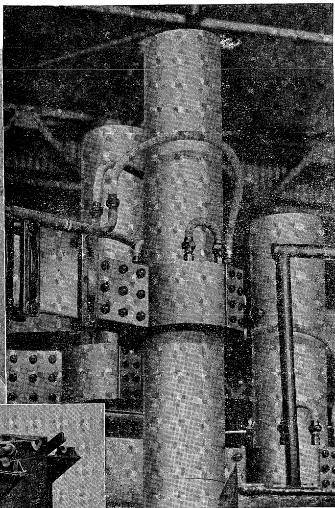
某社納入20吨トツプチャーヂ式弧光爐
