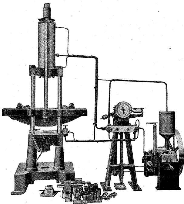
五拾噸 東式 強弱試驗機 檯式萬能材料機
