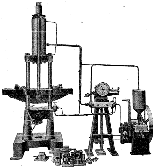
五拾式 東京衡機 強弱試驗機 材料試驗機
