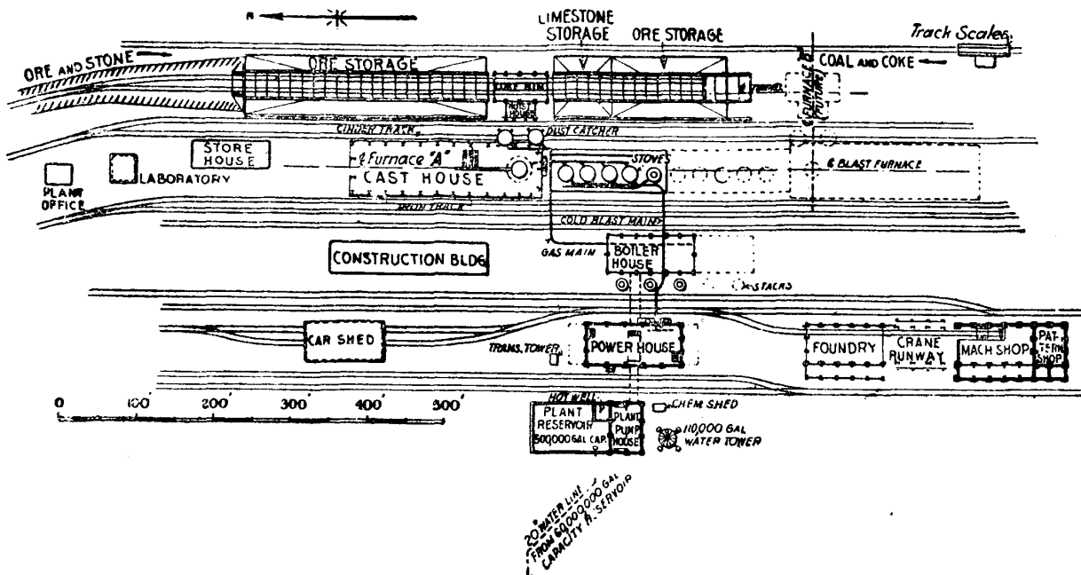
龍煙製鐵所工場の平面圖
