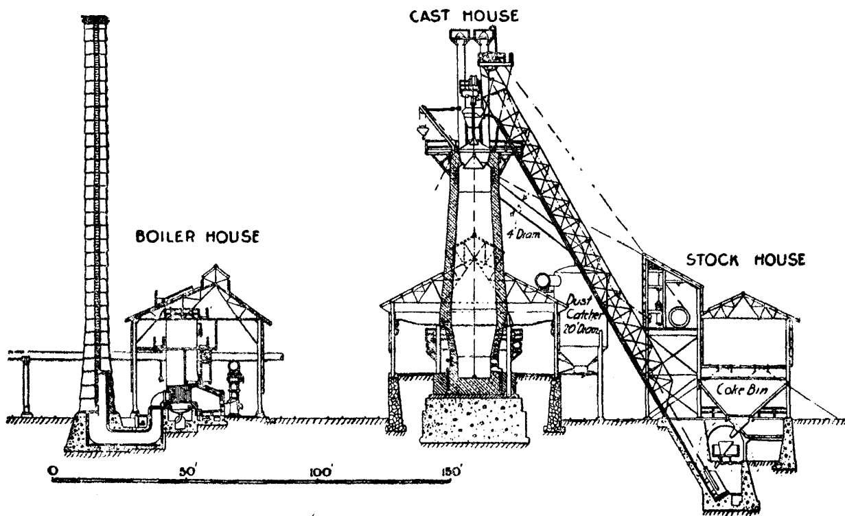
龍煙製鐵所鑄鑪の断面圖
